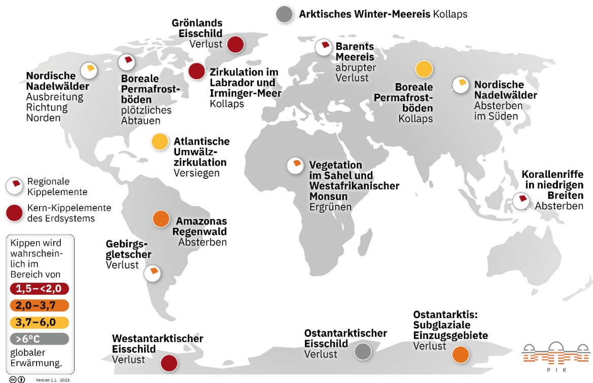
Abbildung 3: Geographische Verteilung der Kippelemente und des Erderwärmungsausmaßes, in dem ihr Auslösen wahrscheinlich wird.
